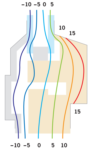
Die Isotherme verlaufen bei den Holz-Metall-Fenstern in einem Bereich, der eine ideale Wärmedämmung garantiert.
